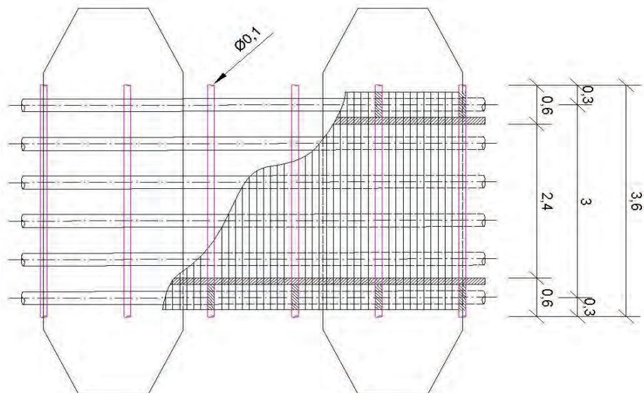
Schemat 1. Schemat konstrukcji pomostu z balustradami
