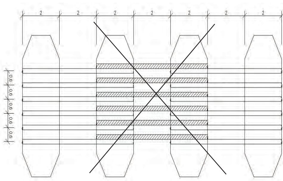
Schemat 2. Zdyskwalifikowane rozwiązanie łączenia katamaranów pomostem pośrednim
