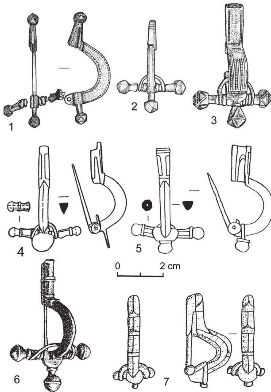
Рис. 3. «Варварские» реплики фибул с «луковичными наверхшими» в низовьях рек Эльбы (1–3) и Вислы (6, 7), в черняховском ареале (4, 5): 1, 2 – Pritzier, тип Leutenkirch и Leipferdingen (Kr. Ludwigslust, Mecklenburg-Vorpommern); 3 – тип Ulm; 4 – Birlad-Valea-Seaca, погр. 342; 5 – Izvoare-Neamt, погр. 10; 6 – бывш. Greibau, Kr. Samland, погр. 56 (найдена среди кальцинированных костей в урне с сосудом-приставкой, янтарной бусиной, с бронзовым кольцом и с железной пряжкой), 7 – Wielbark, погр. 548 (1–3 – по: Voß, 1998a, Abb. 3, 3, 4; Abb. 9, 1, 2; 4, 5; 7 – Kazanski, 1998, fig. 5, 2–6; 6 – Tischler, Kemke, 1902, Taf. V, 19).
