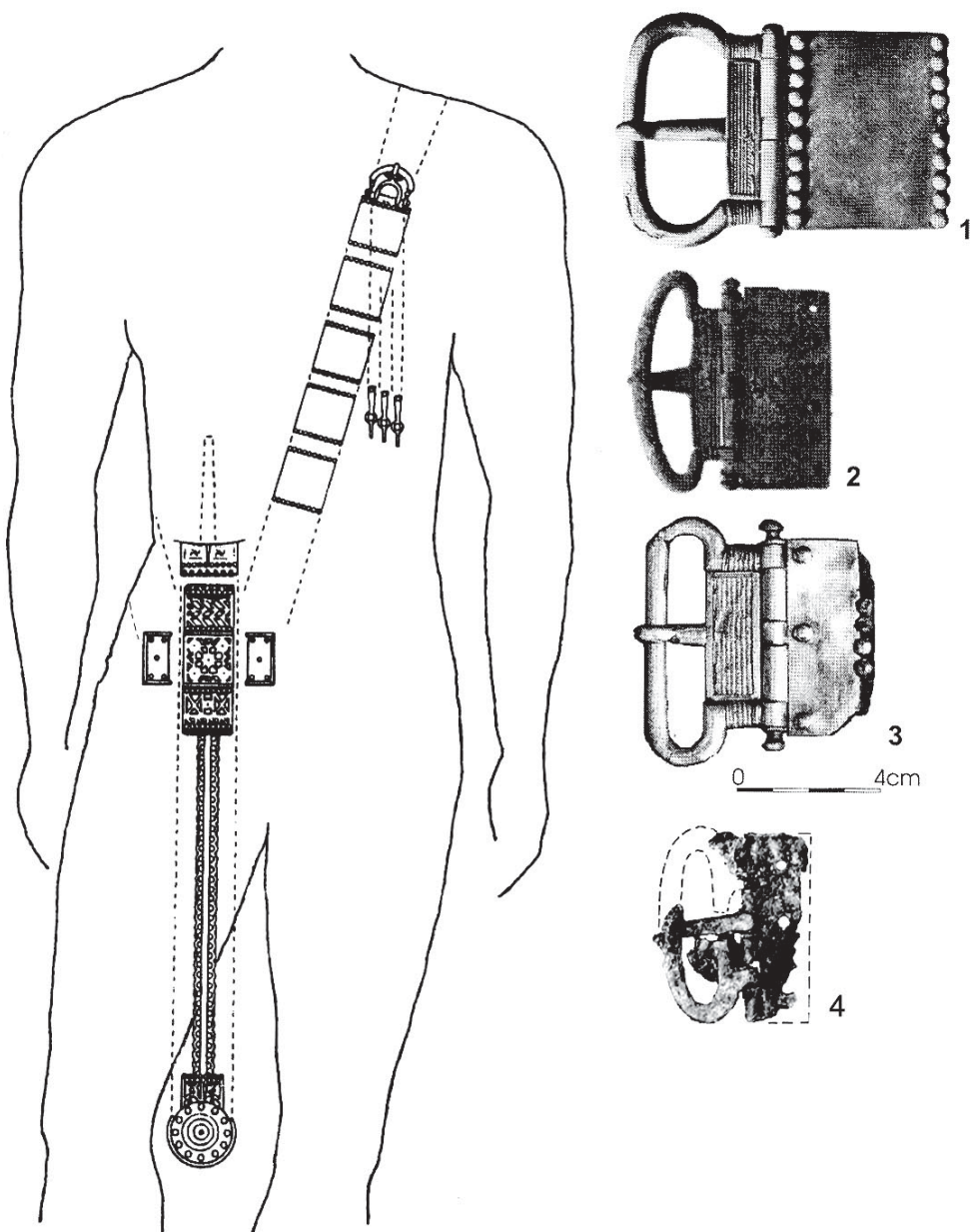
Рис. 7. Римская португья типа balteus (слева – реконструкция К. фон Карнап-Борнхайма и Й. Илкера) и пряжки к ней: 1 – Торсберг, 2 – Стёрлинге, 3 – Йогучай, 4 – Prussia-Museum (по: v. Carnap-Bornheim, Ilkjær, 1996, Tab. 13; 1–3 – Tamulynas, 2005, 4 pav., 4 – фонды КОИХМ).
