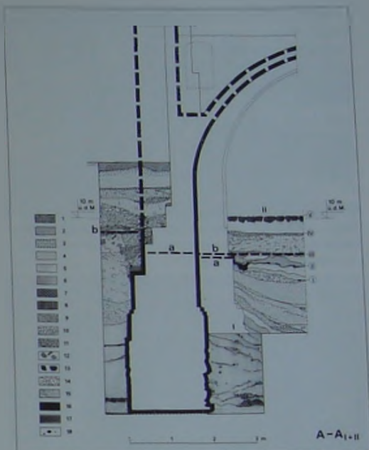
Abb. 9. Schnitt durch das Fundament und die Erdgeschosskonstruktion der Südwand zusammen mit der Zuschüttung von innen und aussen des Gebäudes, sowie Boden (Ziffern in Kreisen). Zeichn. Verfasser.
