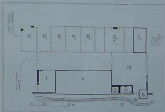
Abb. 5. Rekonstruktionsplan des Karwan-Vorwerks in der Ordenszeit. Mit dicken Linien sind die erhaltene gebliebenen, Bauten bezeichnet. Schwarz sind die nicht existierenden, aber archäologisch bestätigten Mauerwerke. Zeichn. Verfasser.
