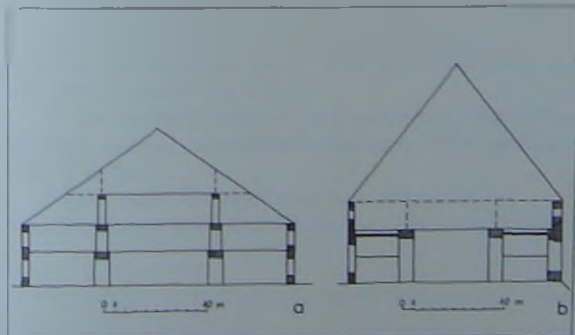
Abb. 15. Die Querschnitte durch a) das Brauhaus zu Doberan b) der Karwan zu Malbork Zeichn. Verfasser.
